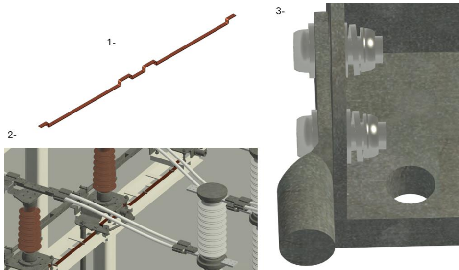
Figura 20 – Exemplo de aplicação prática no modelo de uma família de uso único e outras paramétricas, respetivamente. Legenda: 1- Vista isométrica de um barramento dobrado de forma precisa; 2- Família do barramento aplicada ao modelo da subestação; 3- Terminal de cabo e parafuso com os devidos acessórios, paramétricos que assumem diversas dimensões.
